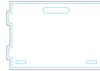
Achterkant lade 4
